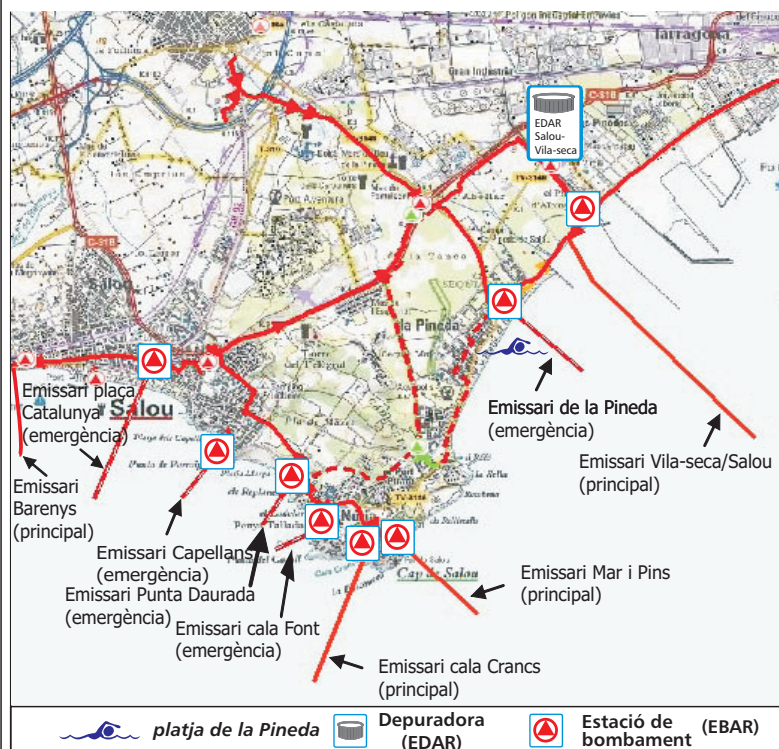
Figura 6. Mapa del sistema de sanejament Vila-seca/Salou
