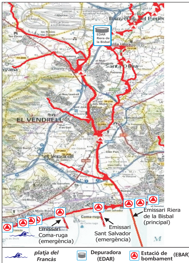
Figura 6. Mapa del sistema de sanejament Riera de la Bisbal
