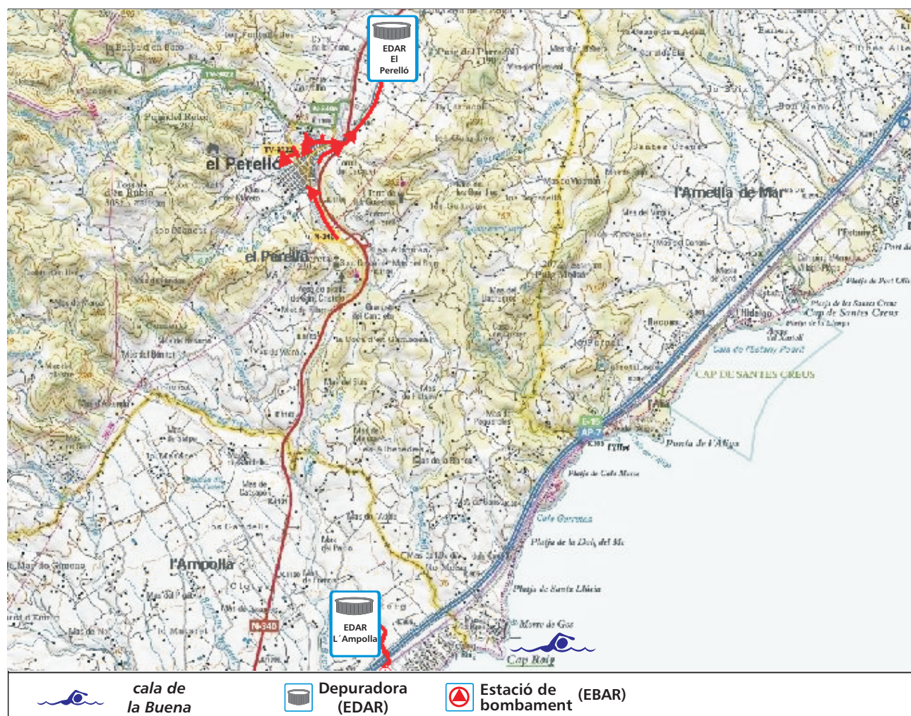
Figura 6. Mapa del sistema de sanejament El Perelló
