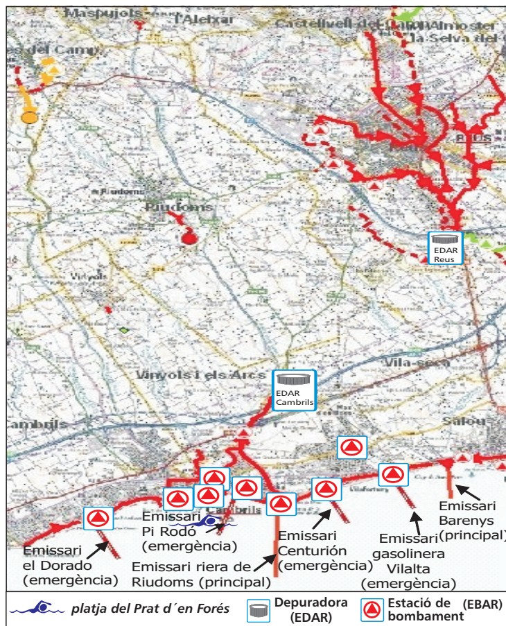
Figura 6. Mapa del sistema de sanejament Cambrils
