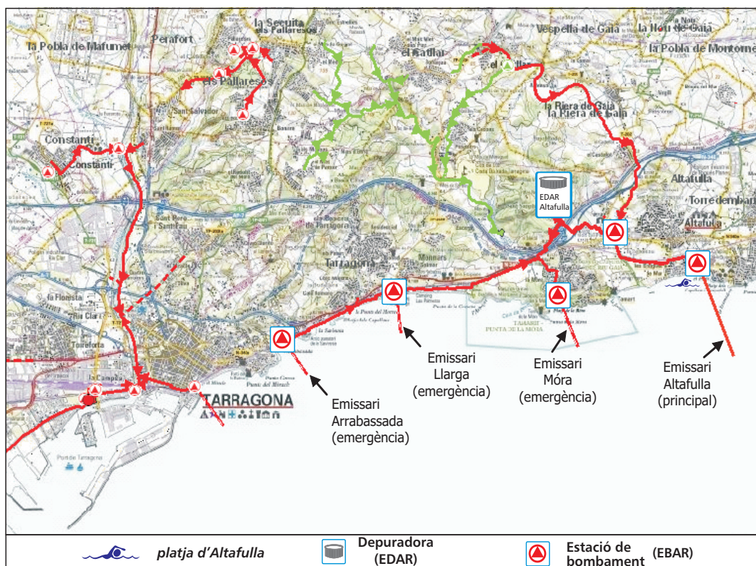
Figura 6. Mapa del sistema de sanejament Altafulla.
