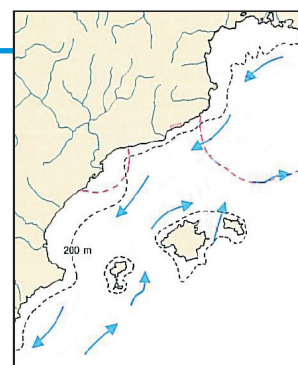
Figura 5. Direcció dels vents principals
