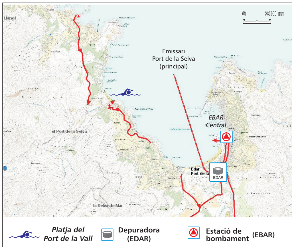
Figura 6. Mapa del sistema de sanejament Port de la Selva
