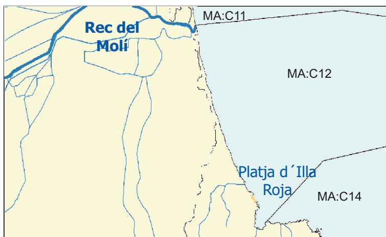
Figura 4. Aports d'aigües superficials i localització de la Massa d'Aigua C12.
