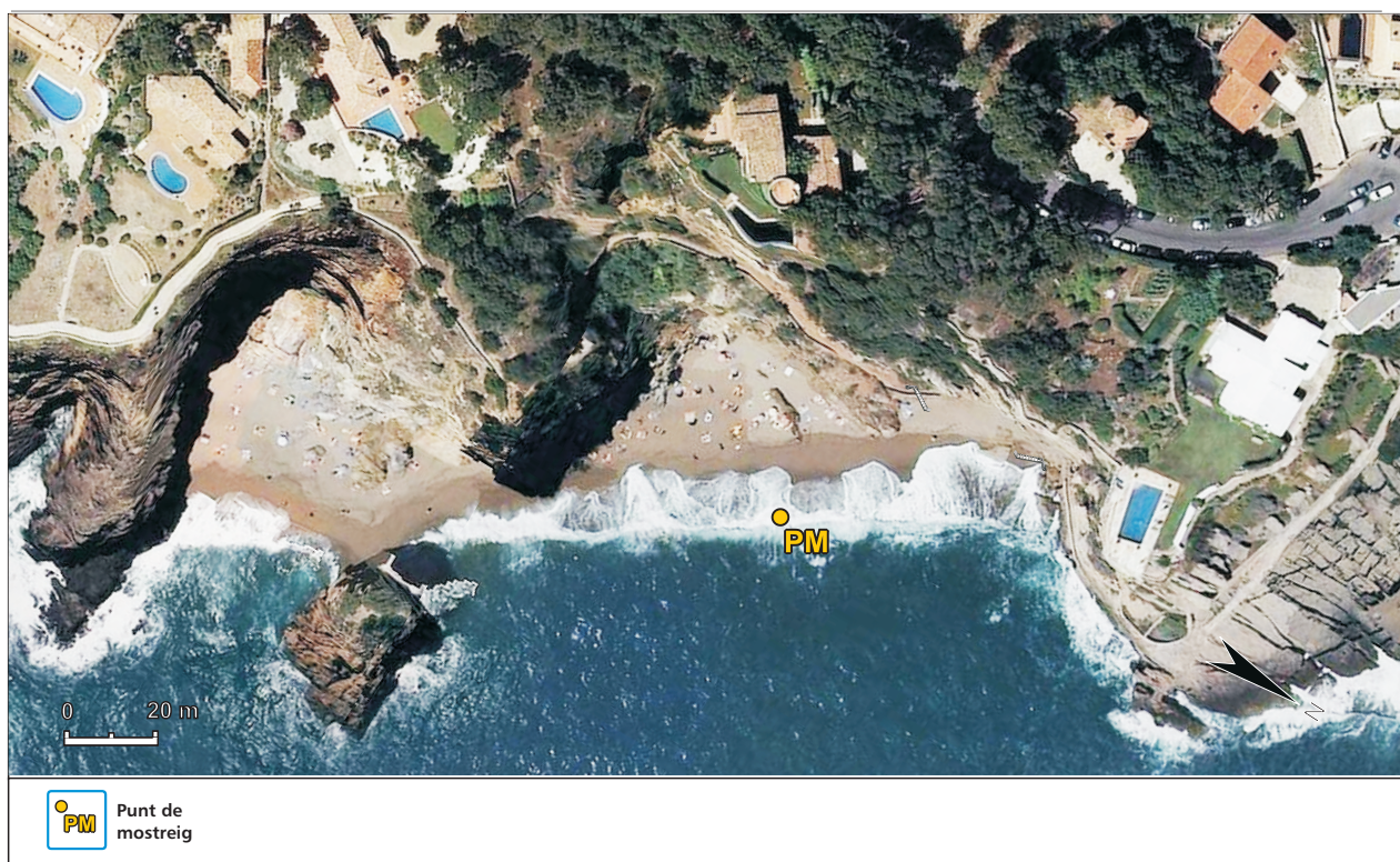
Figura 10. Localització de les sortides potencials d'aigües dolces a la zona de bany.
