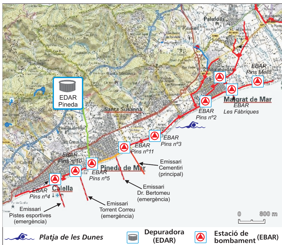
Figura 6. Mapa del sistema de sanejament Maresme Nord.
