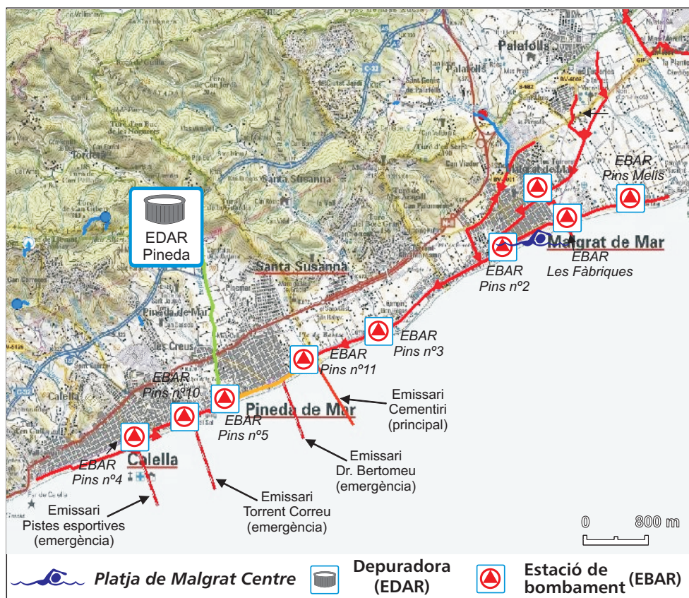
Figura 6. Mapa del sistema de sanejament Alt Maresme.
