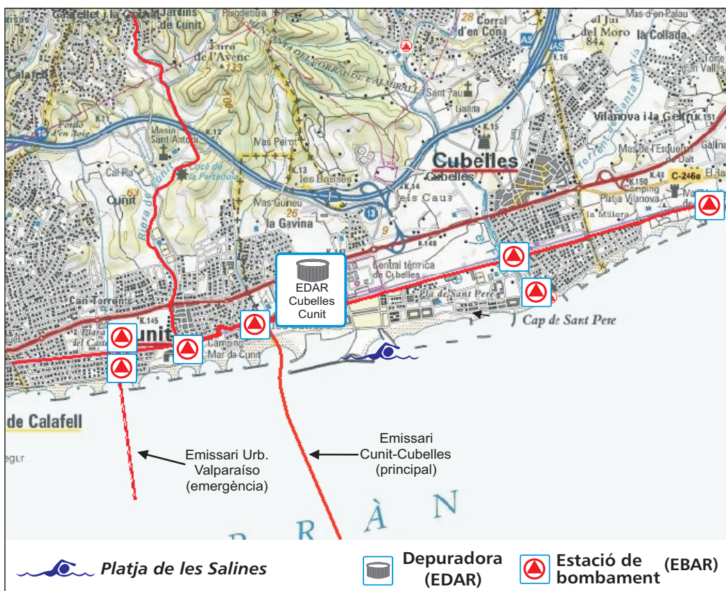
Figura 6. Mapa del sistema de sanejament Cubelles-Cunit.
